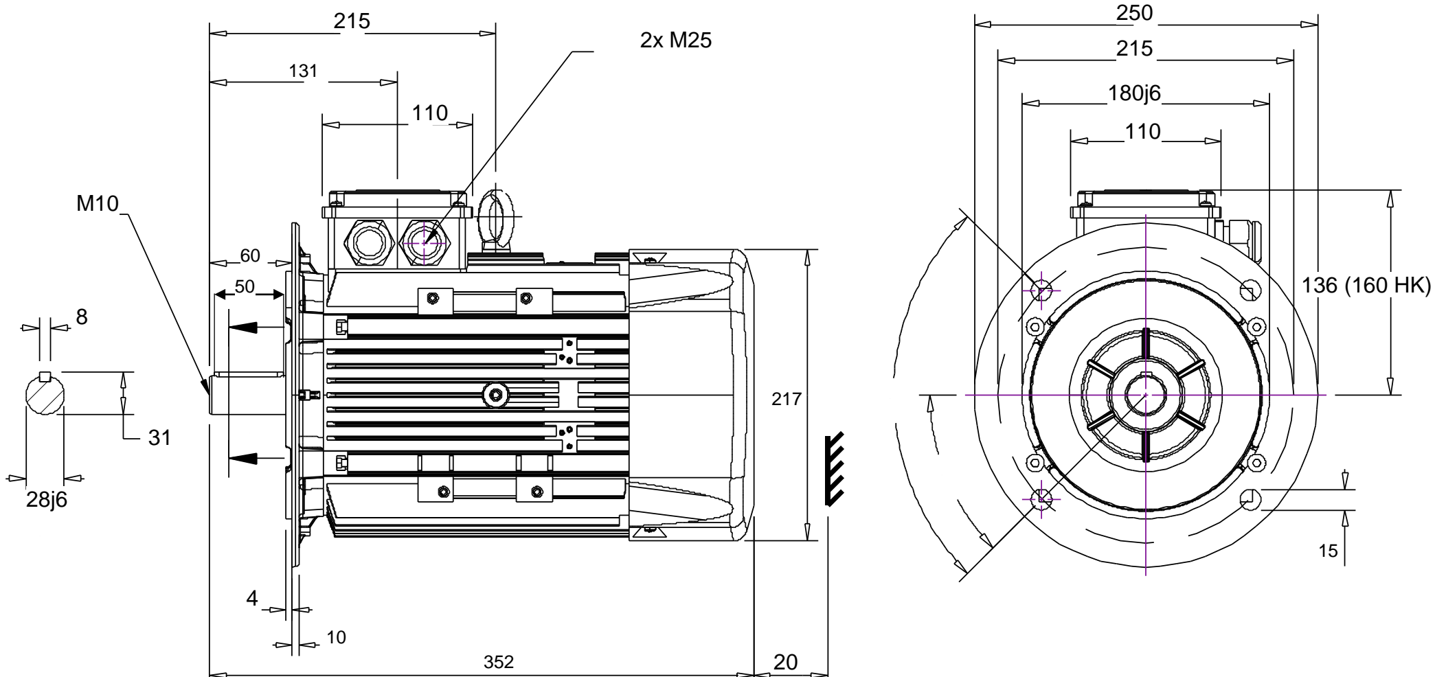
Maßblatt - #34144 - KTE2W 100 L x 4 KT IE2 in Angebot An147206 Position 1
